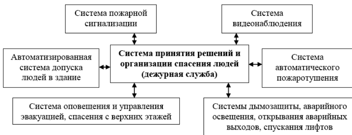
Рисунок 2 – Вариант построения комплексной системы безопасности в здании
